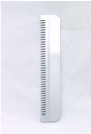
品名:S平面削菜機刀片 (細目) 尺寸:105*19mm
