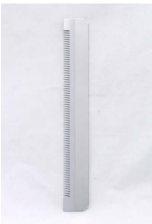
品名:L平面削菜機刀片 (細目) 尺寸:146*19mm
