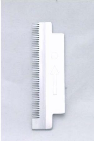
品名:削菜機刀片(細目) 尺寸:64*19mm
