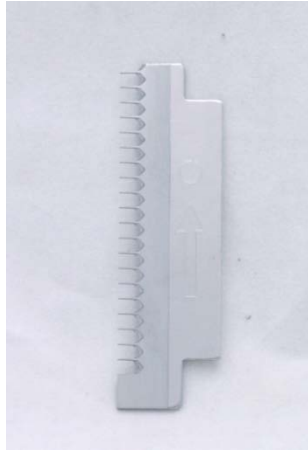
品名:削菜機刀片(中目) 尺寸:64*19mm
